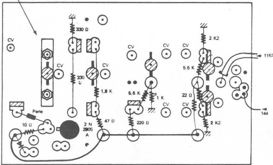
FACE INFÉRIEURE (CÔTÉ MASSE)
