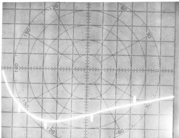
Courbe de 1.6 à 10 MHz.
