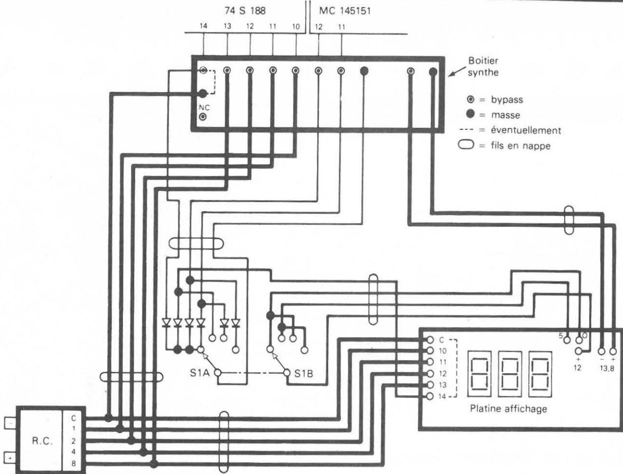
Fig. 6. SCHÉMA D'INTERCONNECTION
