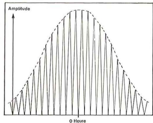
Ces franges révèlent des informations sur la position de la source qui les a produites. Bien entendu, la frange de plus grande amplitude correspond au passage de la radiosource dans le plan médian des antennes. Ces franges représentent en quelque sorte le diagramme de rayonnement complexe de l'interféromètre et en pointillé, celui d'une seule antenne. En laissant l'astre «filer» dans le champ de l'interféromètre, le nombre de franges par heure est proportionnel à l'espacement des antennes en longueur d'onde de travail divisé par quatre, valide pour un astre passant au méridien avec une déclinaison nulle.
