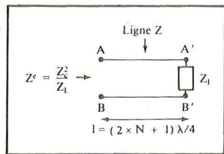
Fig. B.3.4c. Si la ligne mesure électriquement un nombre impair de quart d'ondes, l'impédance à l'entrée est donnée par la formule Z_e = Z_c^2/Z_L .
