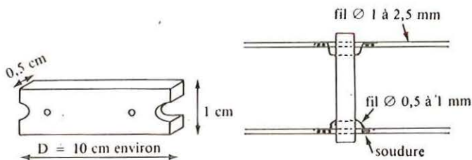
Fig. B.4.4a. Isolateurs à réaliser en matière plastique, lucifex ou plexiglas et méthode de fixation sur les deux fils de la ligne.
