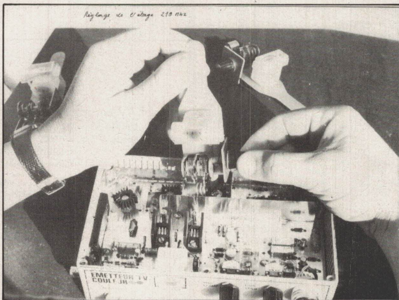
Réglage de l'étage 138,5 MHz à l'aide de l'oscilloscope.
