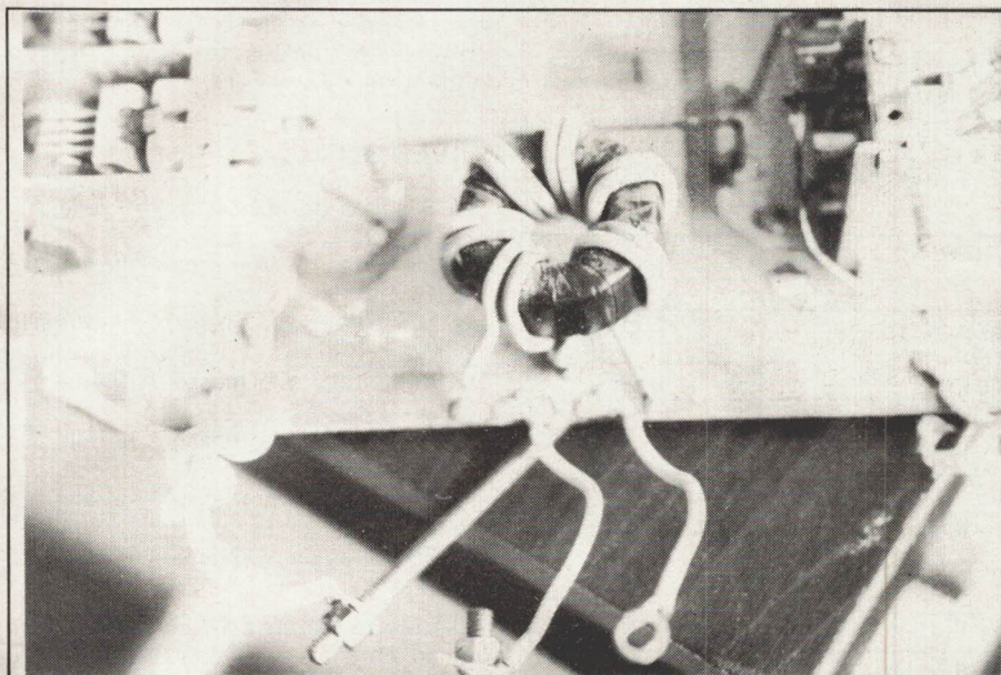
Le montage du tore 4C6.
