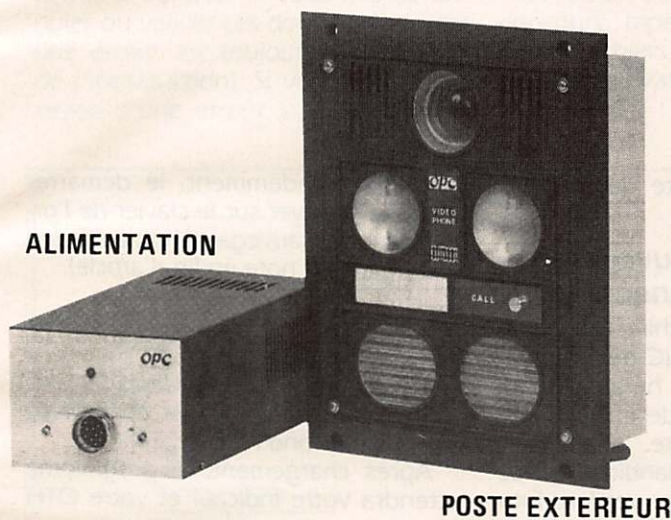
Portier interphone vidéo
