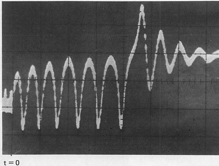
OSCILLOGRAMME N° 4
