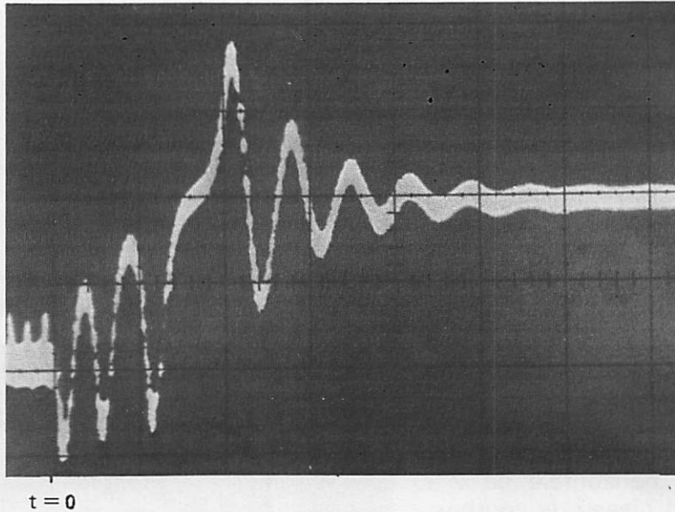
OSCILLOGRAMME N° 3
