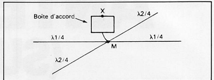
Figure IV. 2.11d. - Des « radians » \lambda/4 disposés tout autour de la prise de terre en améliorant les performances H.F.
