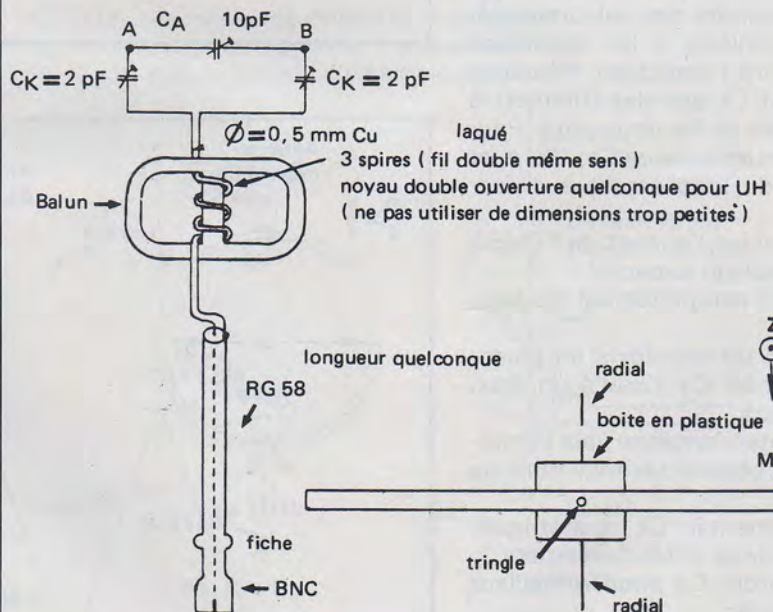
Fig. 15 b.2.1. 2-m-EMBA à couplage capacitif
