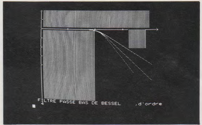
TROISIEME EXEMPLE: BESSEL ORDRE 4 f_0 = 1 \text{ kHz} f_1 = 20 \text{ kHz} A = 40 \text{ db}
