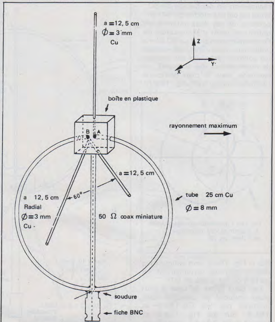
Fig. 15 b.3.1. Autre EMBA 2 m à couplage capacitif ( même vue de dessus que Fig. 15 b.2.2. )
