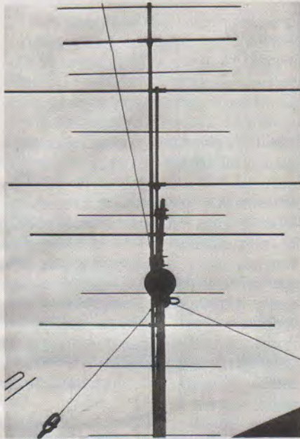
ANTENNES VUES DE DESSOUS 1 - antenne réception 144 MHz (radio) 2 - antenne TV bande 1 - canal E4
