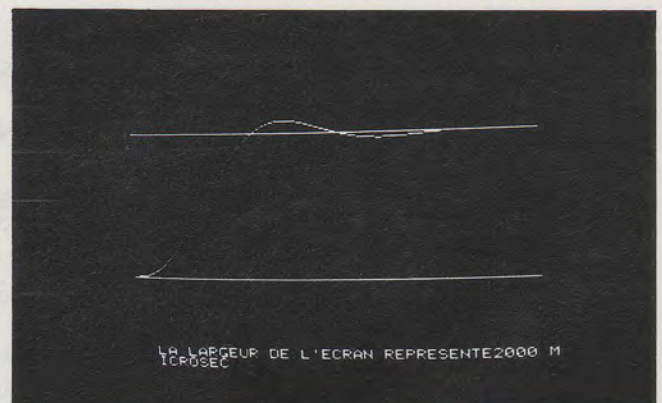
DEUXIEME EXEMPLE: LEGENDRE ORDRE 3 f_0 = 1 \text{ kHz} f_1 = 20 \text{ kHz} A = 40 \text{ db}
