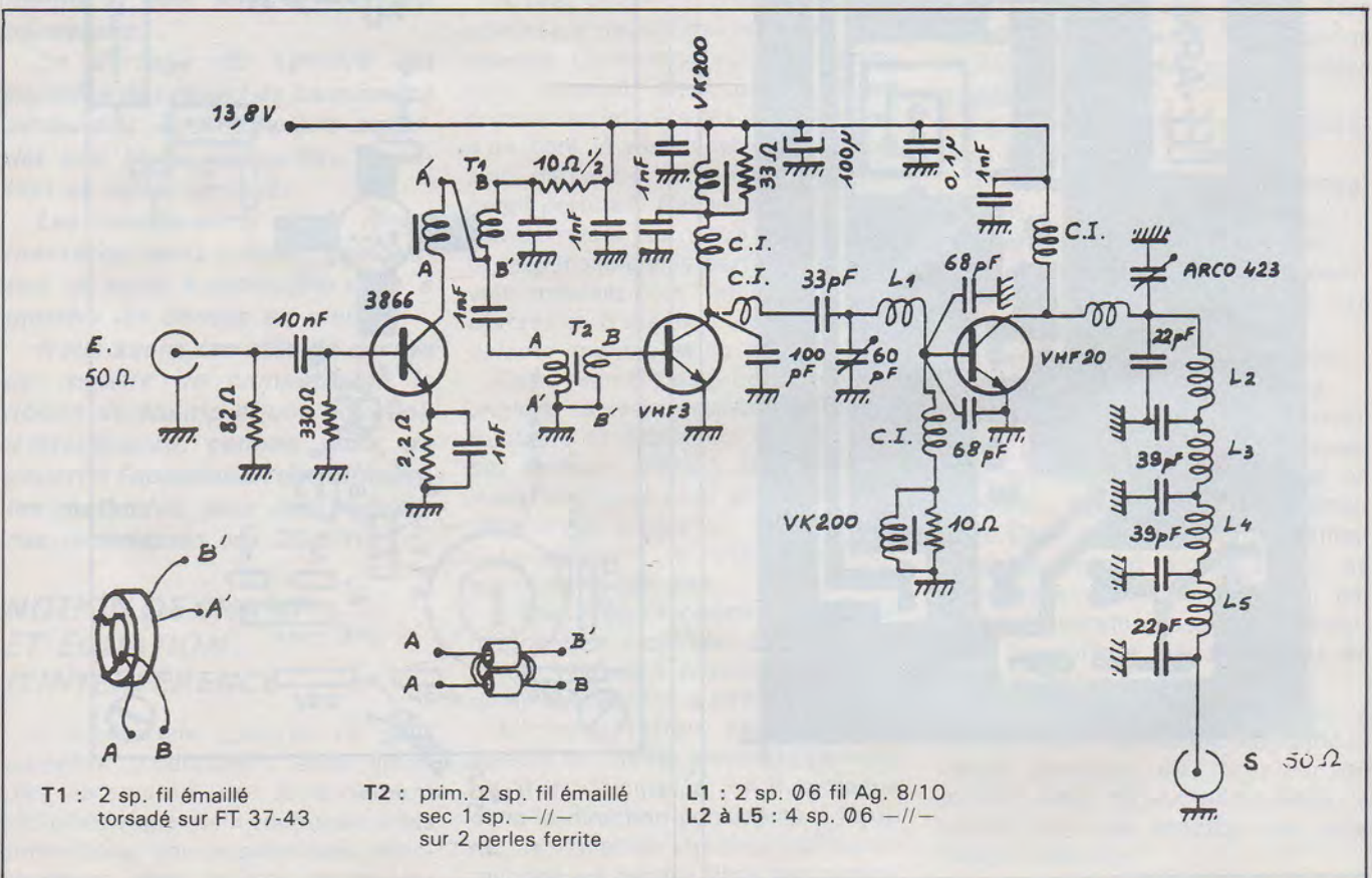
Fig. 1 : APM20 SCHÉMA
