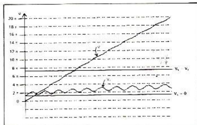
Régime de PULL-OUT F_1 = 63.5 \text{ kHz}
