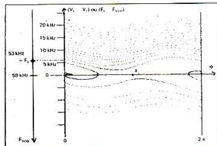
Régime de PULL-OUT F_1 = 59.5 \text{ kHz}
