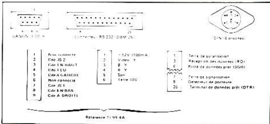
Figure 4 : Schéma de brochage des connecteurs
