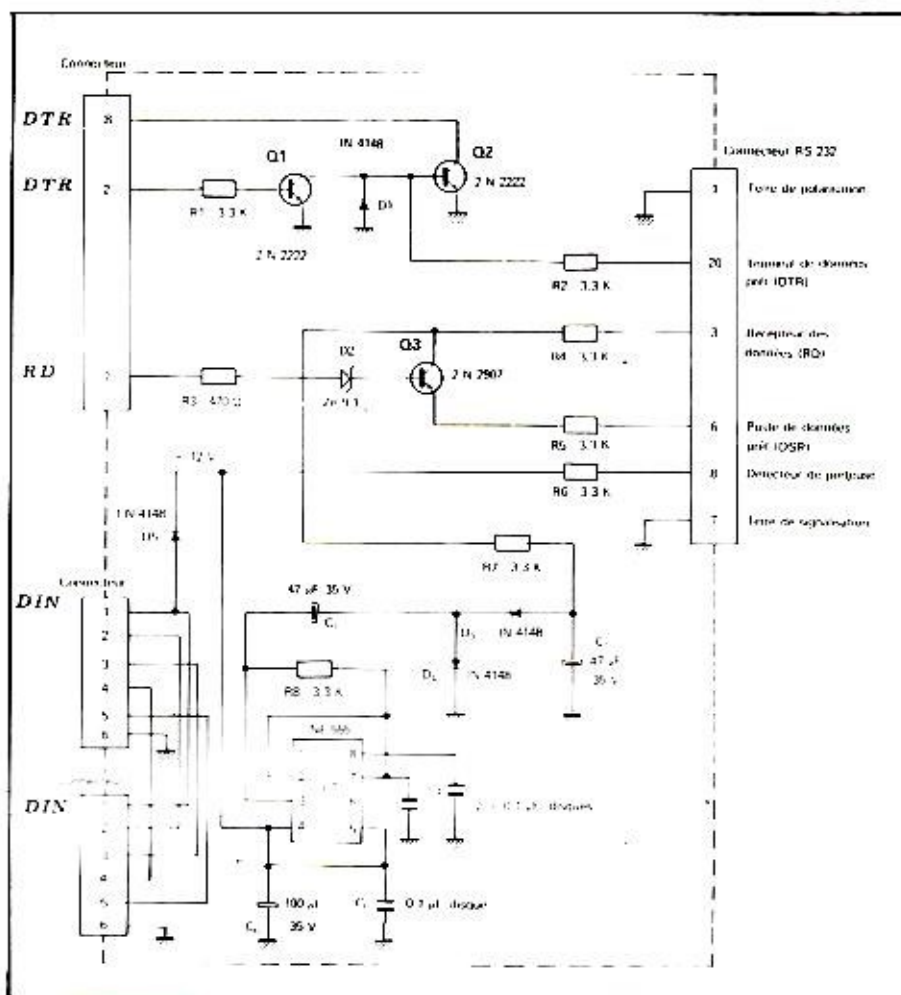
Figure 2 : Schéma électrique
