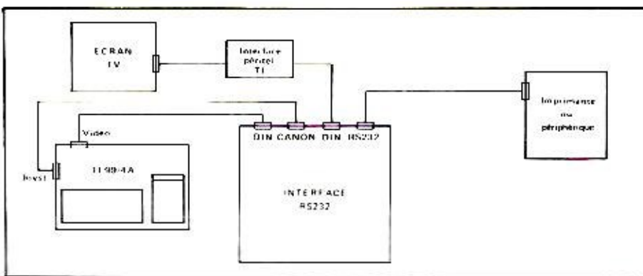
Figure 3: Schéma des liaisons
