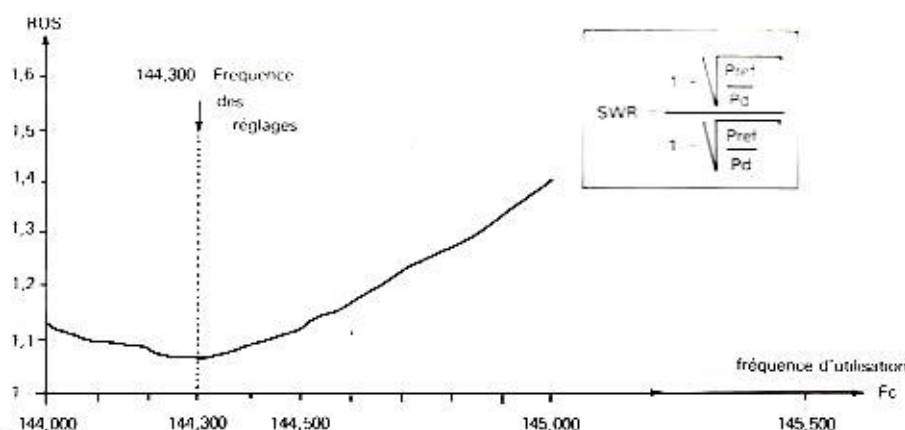
Courbe du ROS - 18 él.
