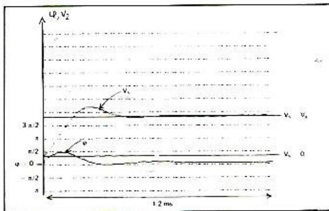
Régime de PULL-OUT F_1 = 58 \text{ kHz}
