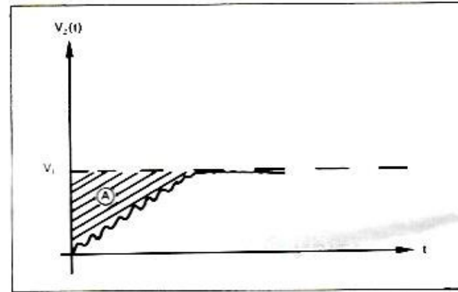
L'examen de V_2(t) , puis la mesure de la surface (A), permet d'évaluer la valeur de \phi .
