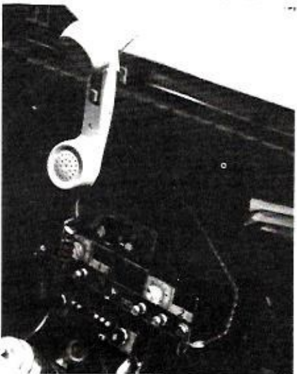
Matériel radio 85 et 160 MHz du véhicule PC de la Croix-Rouge.
