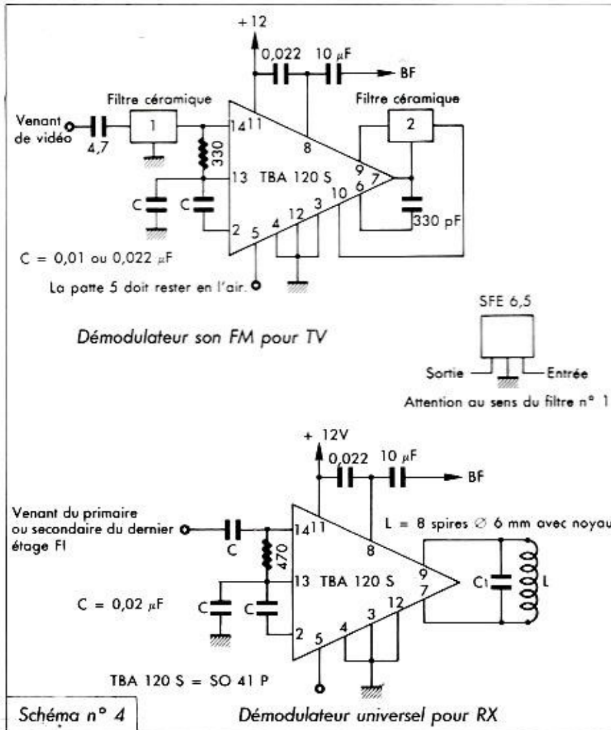
1- Version TU avec filtres céramiques
