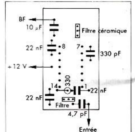
1- Version TU avec filtres céramiques
