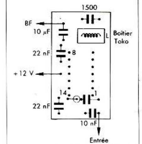
2- Version universelle avec self coïncidence
