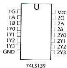
74LS139
