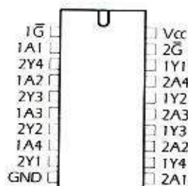
74LS244
