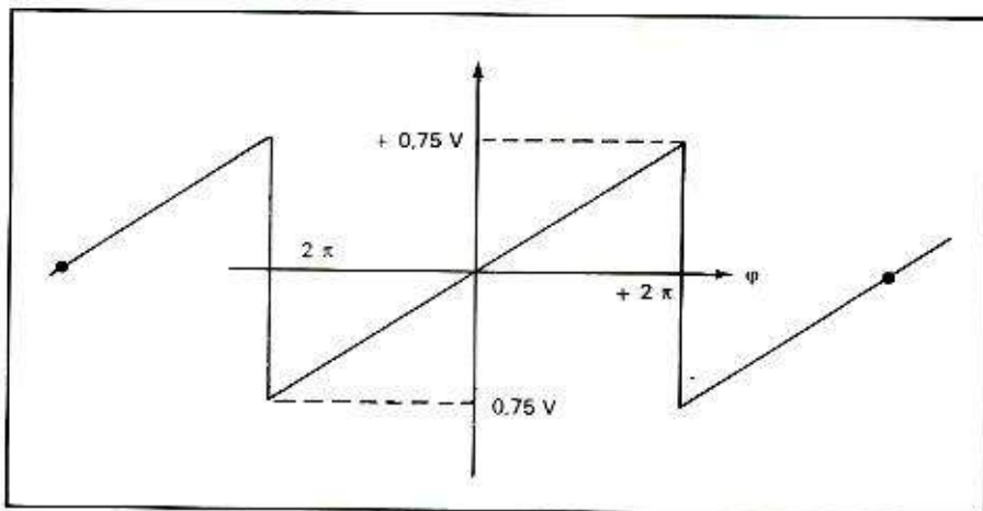
FIGURE 10 Variation de la tension moyenne de sortie.
