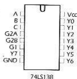
74LS138
