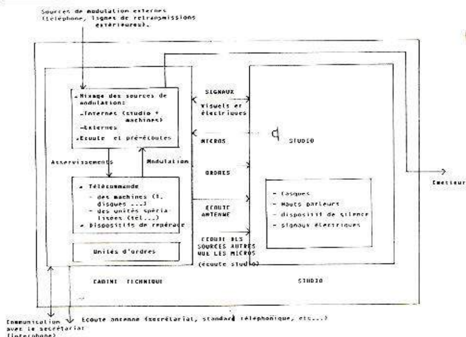
Figure 2 Système complet "studio-technique"
