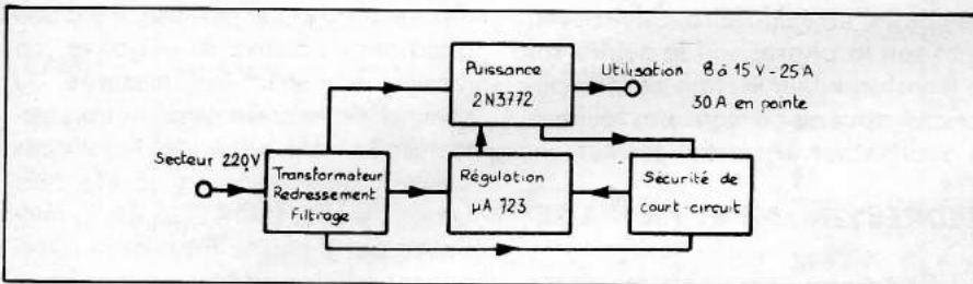
Schéma synoptique de l'alimentation.
