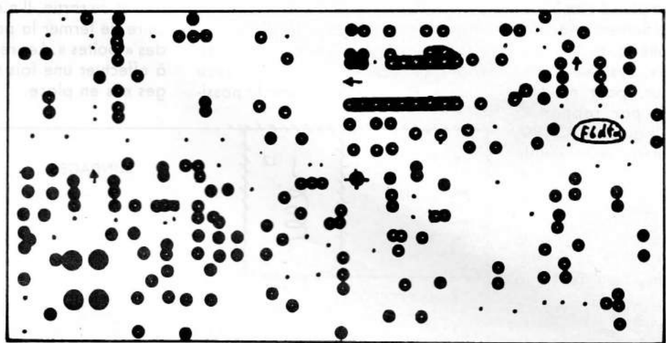
TALKY-WALKY - TDA 7000 Circuit imprimé - vue de dessus
