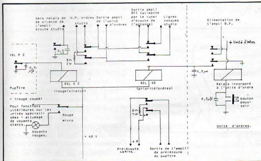
Figure 15 Dispositif rouge/silence/ordres de l'armoire de relais (note : relais tous vus en position repos).
