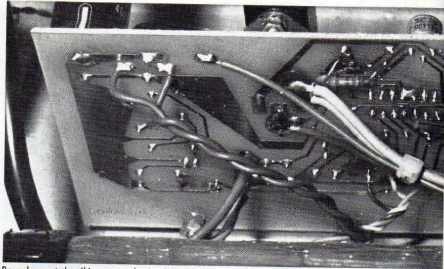
Branchement des éléments sur le circuit imprimé.
