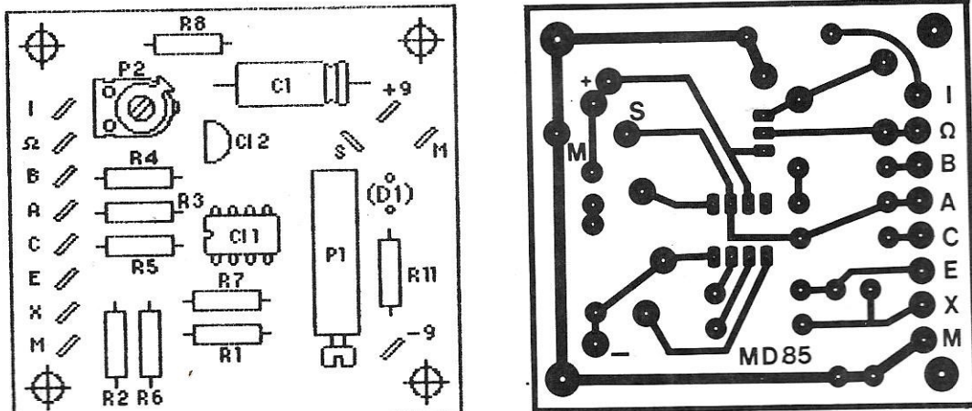
Figure 2 Le circuit imprimé est représenté grandeur nature.
