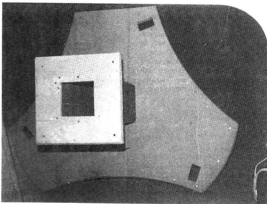
Photo n° 4 Détail du passage des câbles. Les câbles destinés au pupitre passent par une goulotte fixée à l'extérieur entre les deux trous (cette goulotte n'est pas encore fixée ici). Les câbles des micros sortent par le trou du bas (en haut sur la photo). Les câbles d'alimentation des boîtiers casques passent par des petits tubes plastiques d'électricien.
