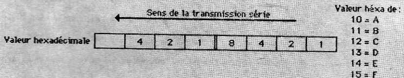
Figure 5 : Organisation du code ASCII
