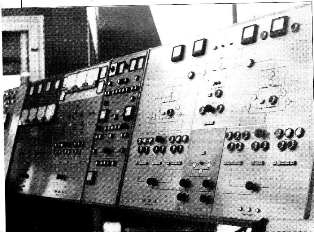
Baie synoptique de contrôle.
