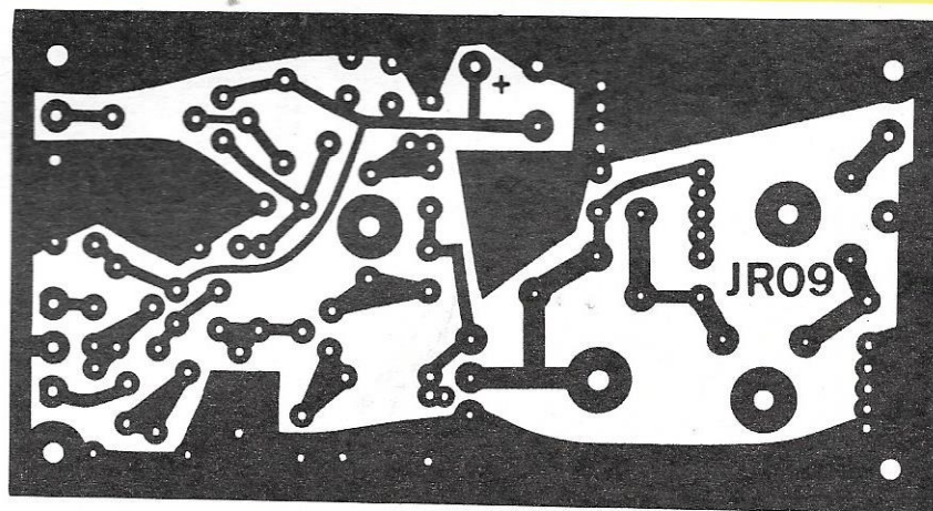
Circuit imprimé JR09, vu côté cuivre, éch. 1/1
