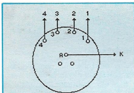
Figure 2 : Câblage du commutateur de changement de fréquence avec le câble plat.
