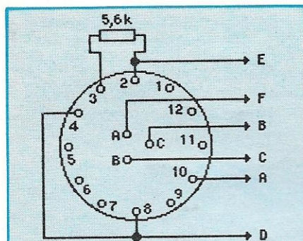
Figure 3 : Câblage du commutateur Sinus/Triangle/Carré avec le câble rond.
