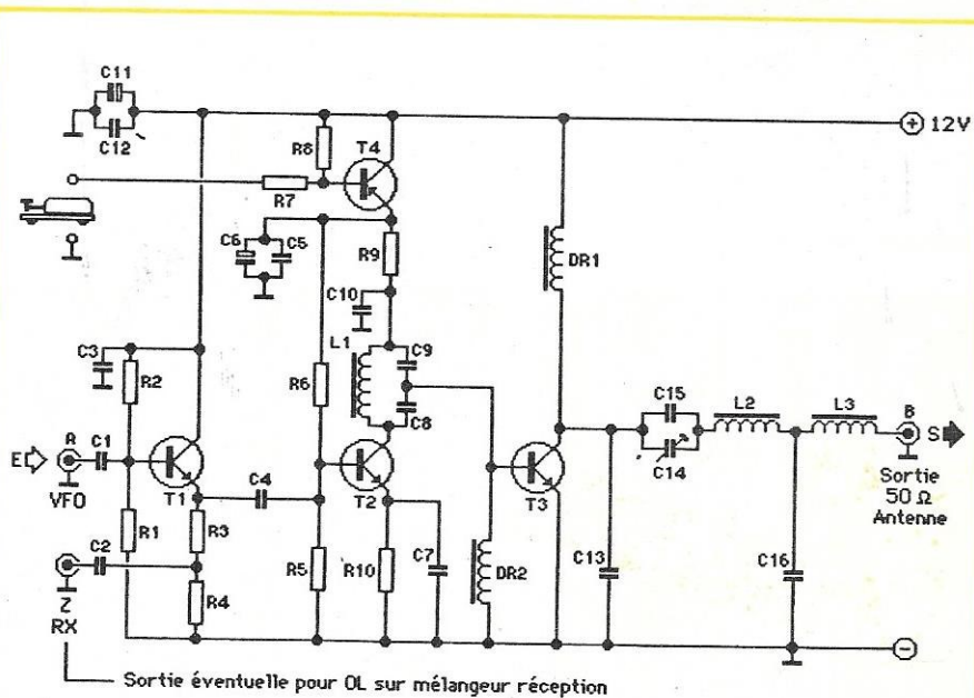
TX JR09 - Schéma partie émission - PA 2W - Sortie HF
