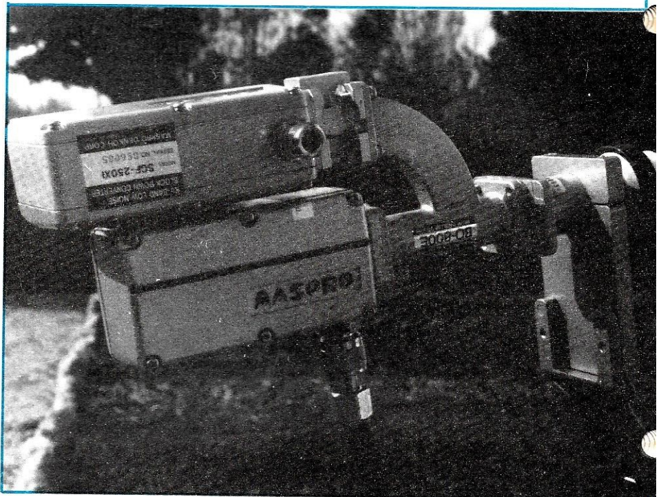
Tête MASPRO : SCE 750X pour ECS-SCF 250x1 : pour Télécom 1 + orthocoupleur + FEED.
