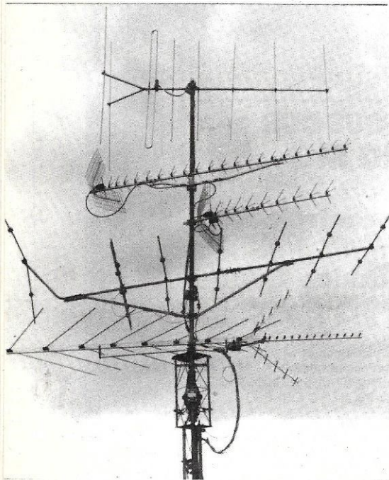
Système antennaire orientable chez Pierre GODOU.
