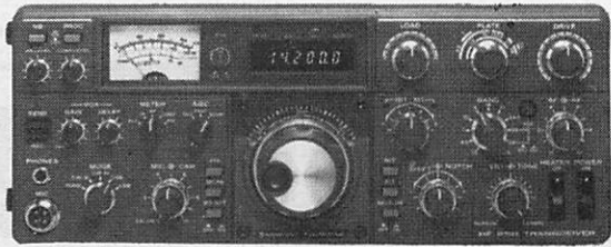
Transceiver bandes amateurs TS 830 S USB - LSB - CW/100 WHF CW-220 W PEP-tubes au final/En Rx : 2 FI-IF shift - VBT - Notch/Alim. secteur incorporée.
