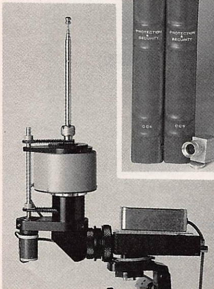
Dispositif émetteur vidéo, télécommande et antenne de voiture dans laquelle la caméra est dissimulée.
