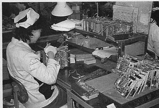
Insertion des sous-ensembles dans les boîtiers.
