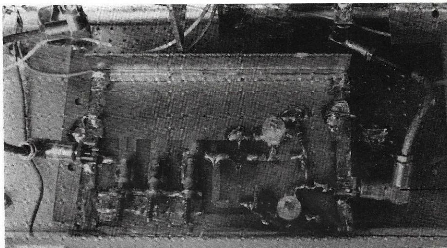
Photo 14 Vue détaillée du tripleur 378/1136
