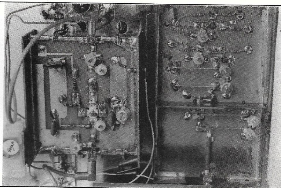
Photo 10 Implantation de la chaîne multiplicatrice
