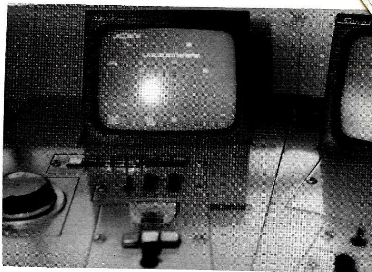
Ecran de contrôle permettant la vérification des plans de vol avant l'établissement des strips.
