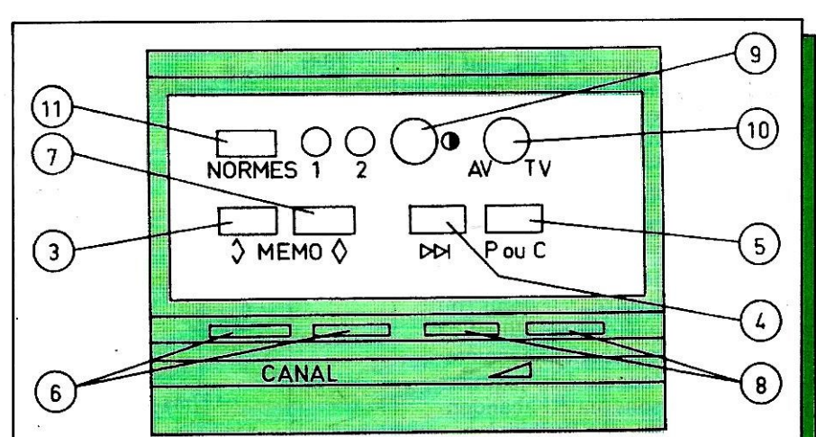
Figure 4 Tableau de commande des nouveaux téléviseurs multistandards Philips
