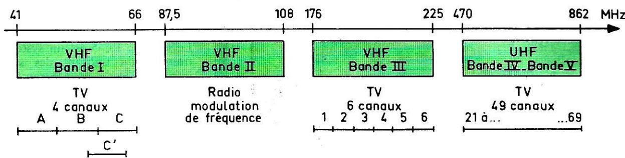
Figure 3 : Bandes de fréquences utilisées en France pour la télévision
