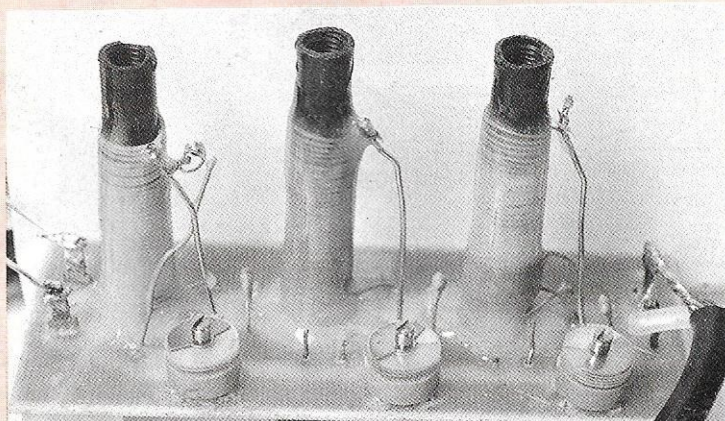
PHOTO 4 - Filtre de bande JR11
