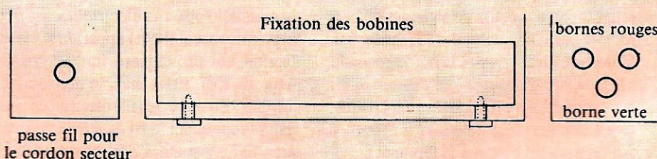
Schéma de montage des bobines.
