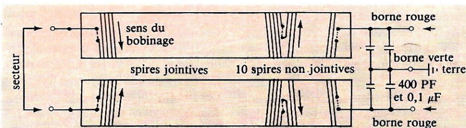
Schéma de montage des bobines.
