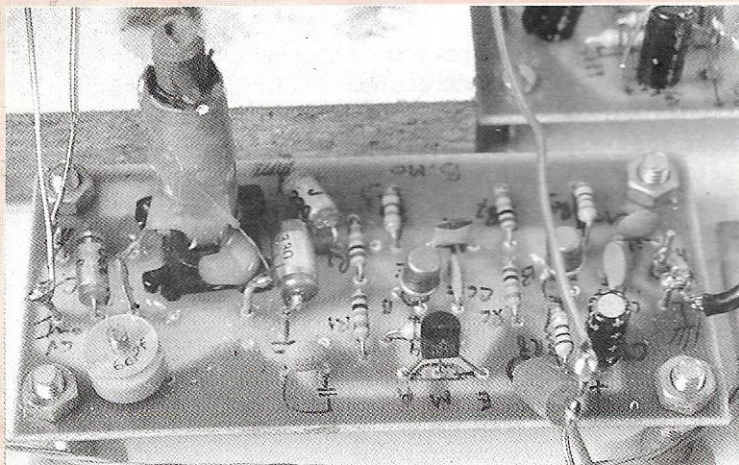
PHOTO 3 - Oscillateur VFO JR02
