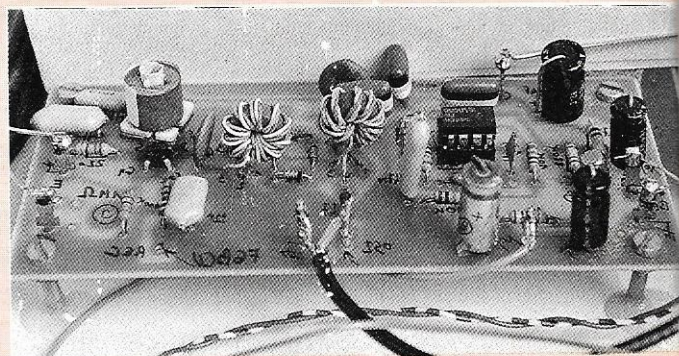
PHOTO 5 - Mélangeur-amplificateur JR08
