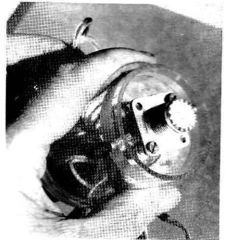
Le montage de la prise SO 239
