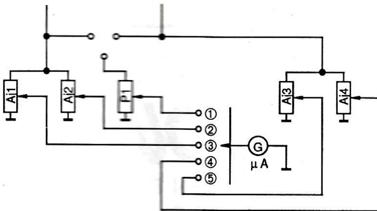
Figure 5 : Utilisation en wattmètre
