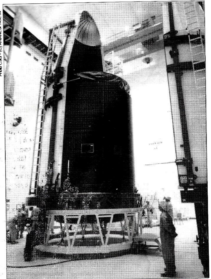
Fermeture de la coiffe sur le satellite Intelsat VI (F.2)
