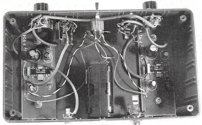
Vue sur le câblage. Rien de bien compliqué.
