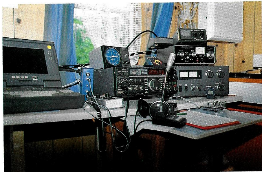
L'installation du matériel de gauche à droite: l'ordinateur portable, la boîte de dérivation BF, le lanceur d'appel, l'IC765, le TL922, la boîte d'accord VHF et le TOS wattmètre Daiwa.
