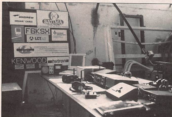
La station EME à l'intérieur du local de la SFM. De g. à d. : Cde antennes, ordinateur, transverter, TS440S et PS430 Kenwood, manip. électronique, filtre BF. Au fond : câble Andrew LDF 7/50, wattmètre et ampli.
