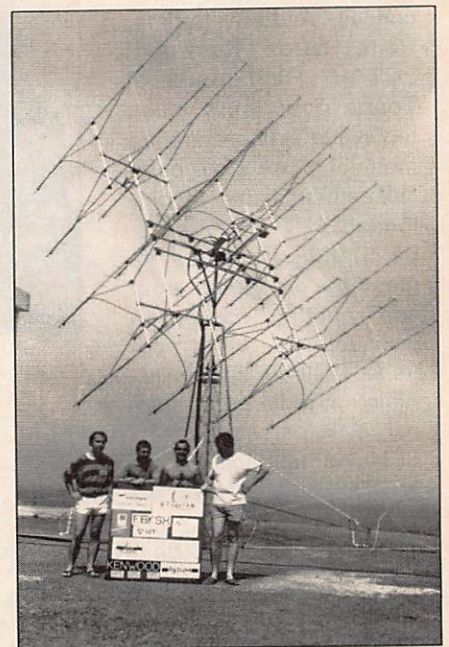
Aériens EME 432 MHz. 1ère partie de l'expédition. De g. à d. : F6EZV, F6CTW, F6HKA et F1EHN.
