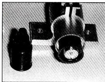
Photo 3 La prise SO239 et son capuchon. Remarquez la pièce de fixation.
