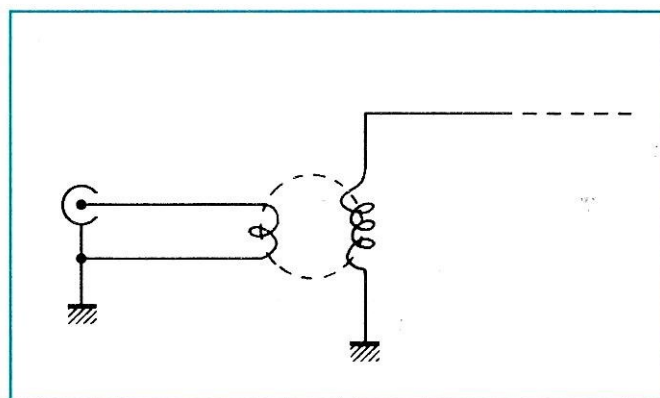
Figure 14 : Adaptation d'impédances apériodique à tore ferrite. Une valeur de compromis sur les nombres de spires permet souvent de fonctionner sur plusieurs bandes, antenne chargée ou non.
