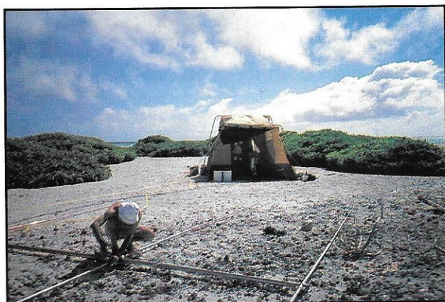
Montage d'une beam sur le site CW.
