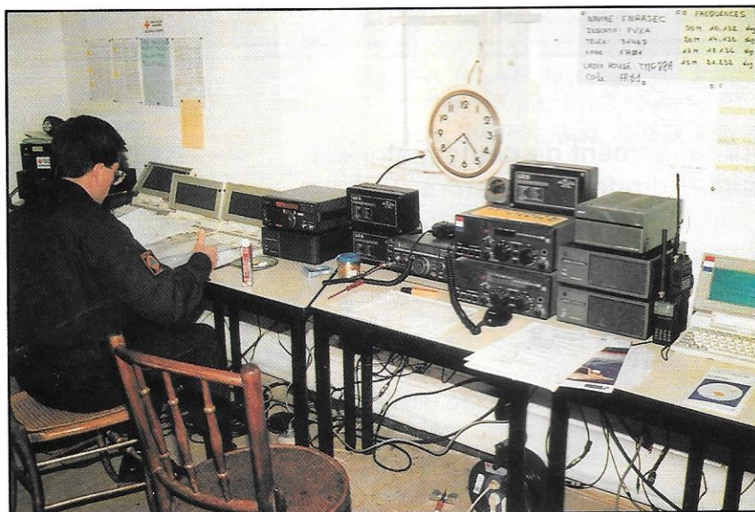
Vue d'ensemble de la station FNRASEC, YOØPCT.
