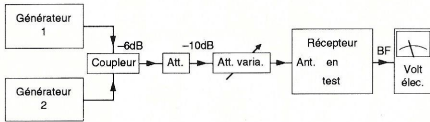
Mesures sur un récepteur
