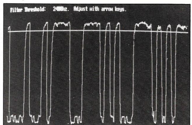
Le réglage de seuil en CW.
