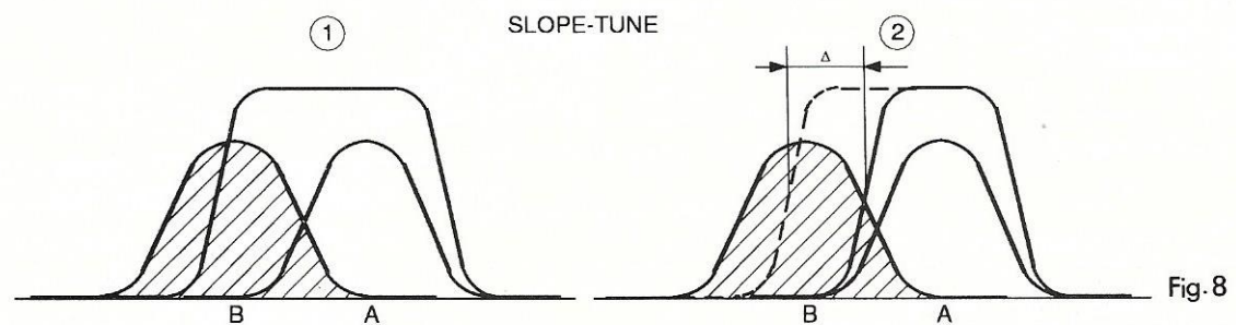
En (2), on diminue considérablement la gêne apportée par le signal B en réduisant la bande passante de la valeur \Delta .
