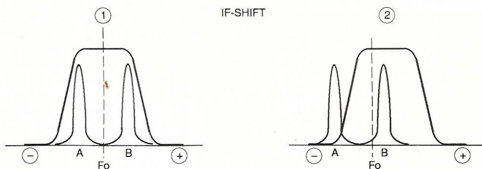
En décalant la FI vers les fréquences plus élevées, on élimine le signal A.
