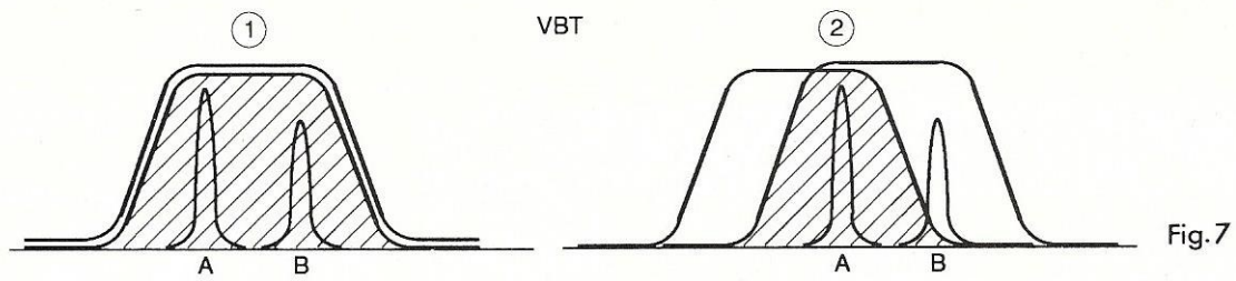
En décalant le filtre variable vers le bas, le signal B n'est plus gênant
