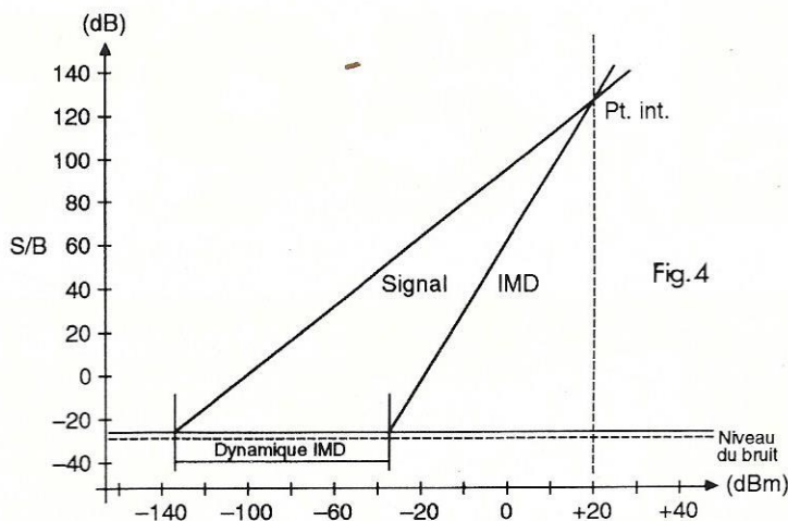
Représentation graphique du point d'interception du 3ème ordre
