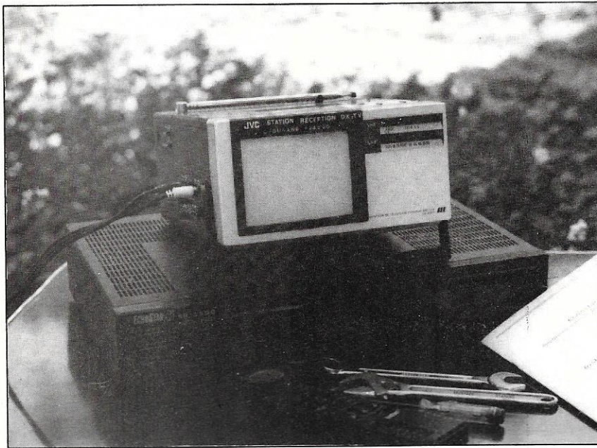
Photo 2 : Le système extérieur d'aide et de contrôle du positionnement de l'antenne. En fait, l'équivalent de la station intérieure avec un TV portatif !
