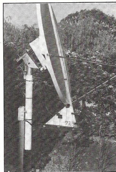
Photo 6 : Réglage de la déclinaison de la parabole en position d'apogée (ici, déclinaison trop importante).
