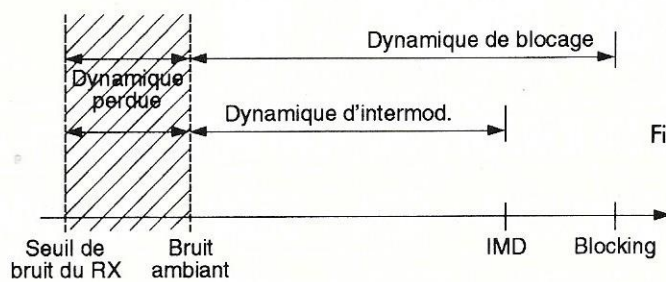
Mesures sur un récepteur
