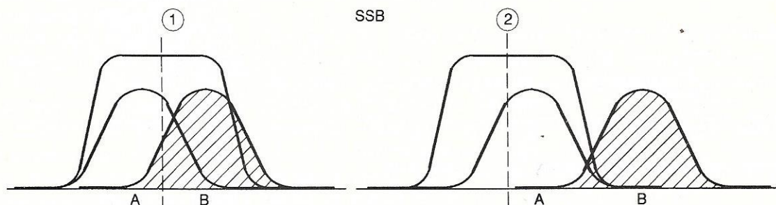
En décalant la FI vers les fréquences plus élevées, on élimine le signal A.
