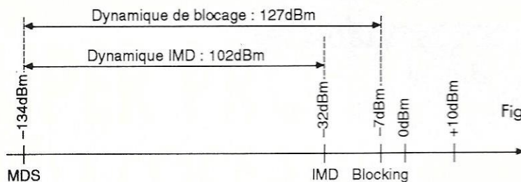
Récepteur XYZ en test, sans préampli
