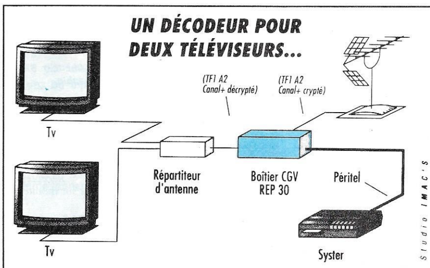
Le principe de connexion de plusieurs récepteurs à un seul décodeur.
