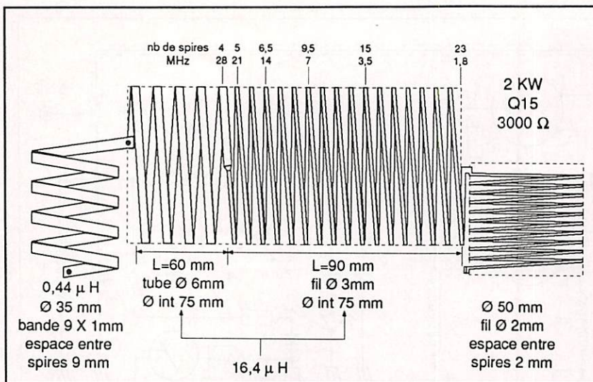
Circuit en π n° 1 pour PA version "A".
