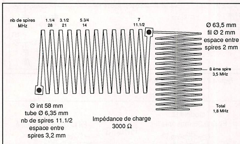
Circuit en π n° 2 pour PA version "B".
