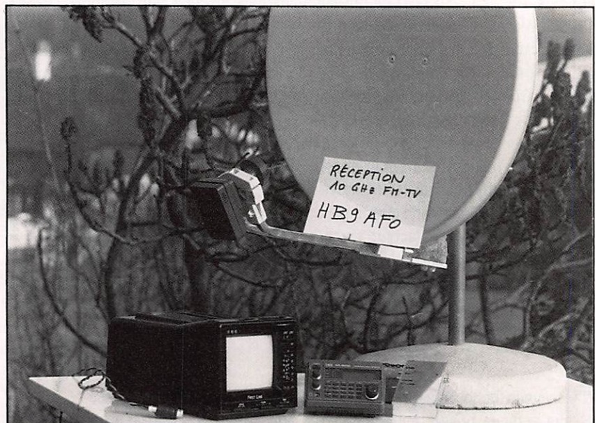
L'ensemble de réception 10 GHz complet.
