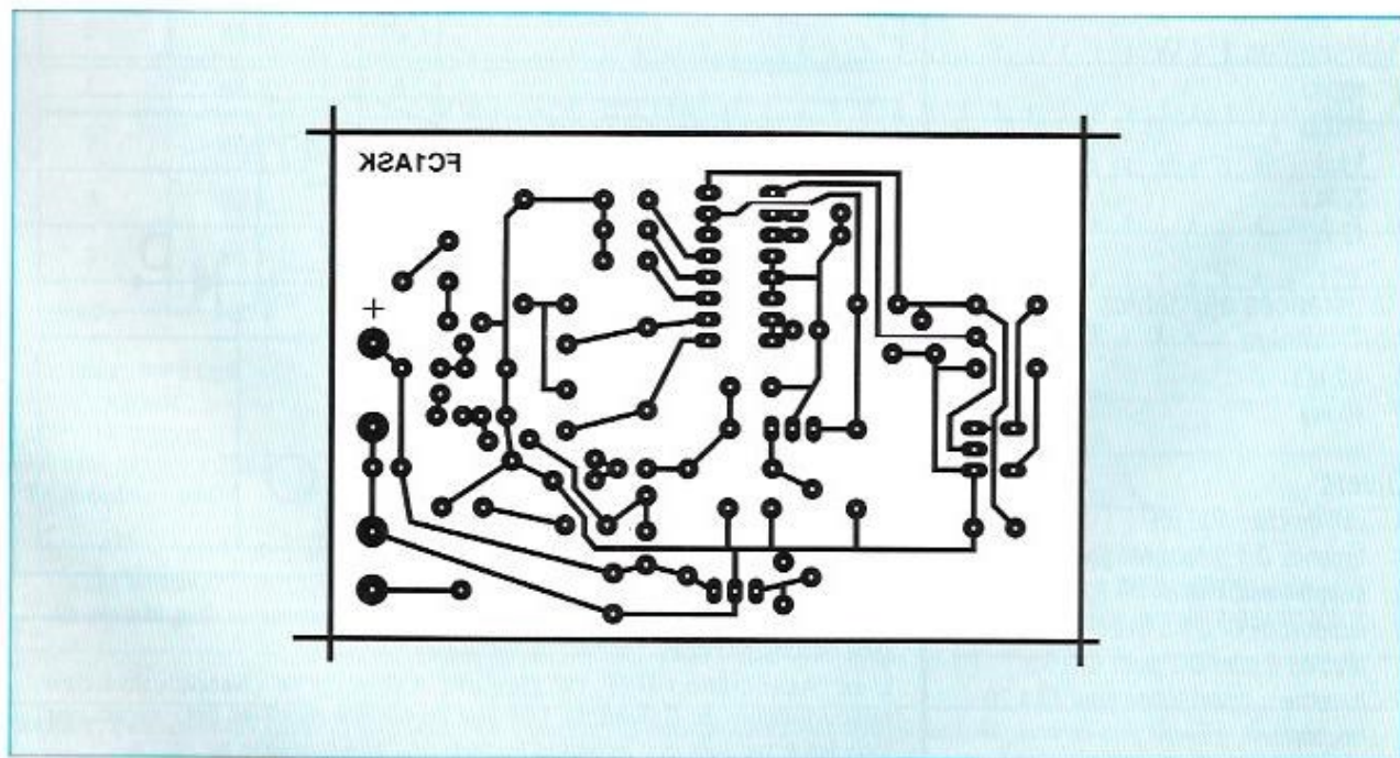
Dessin du circuit imprimé à l'échelle 1
