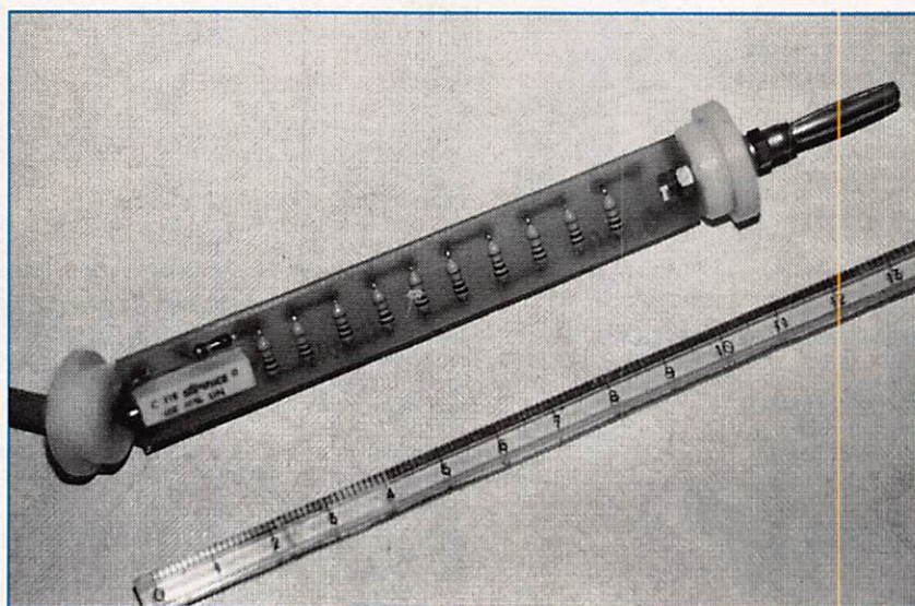
Vue générale de la sonde HT. Sur cette photo, on peut juger sa taille. Le tube isolant est retiré.
