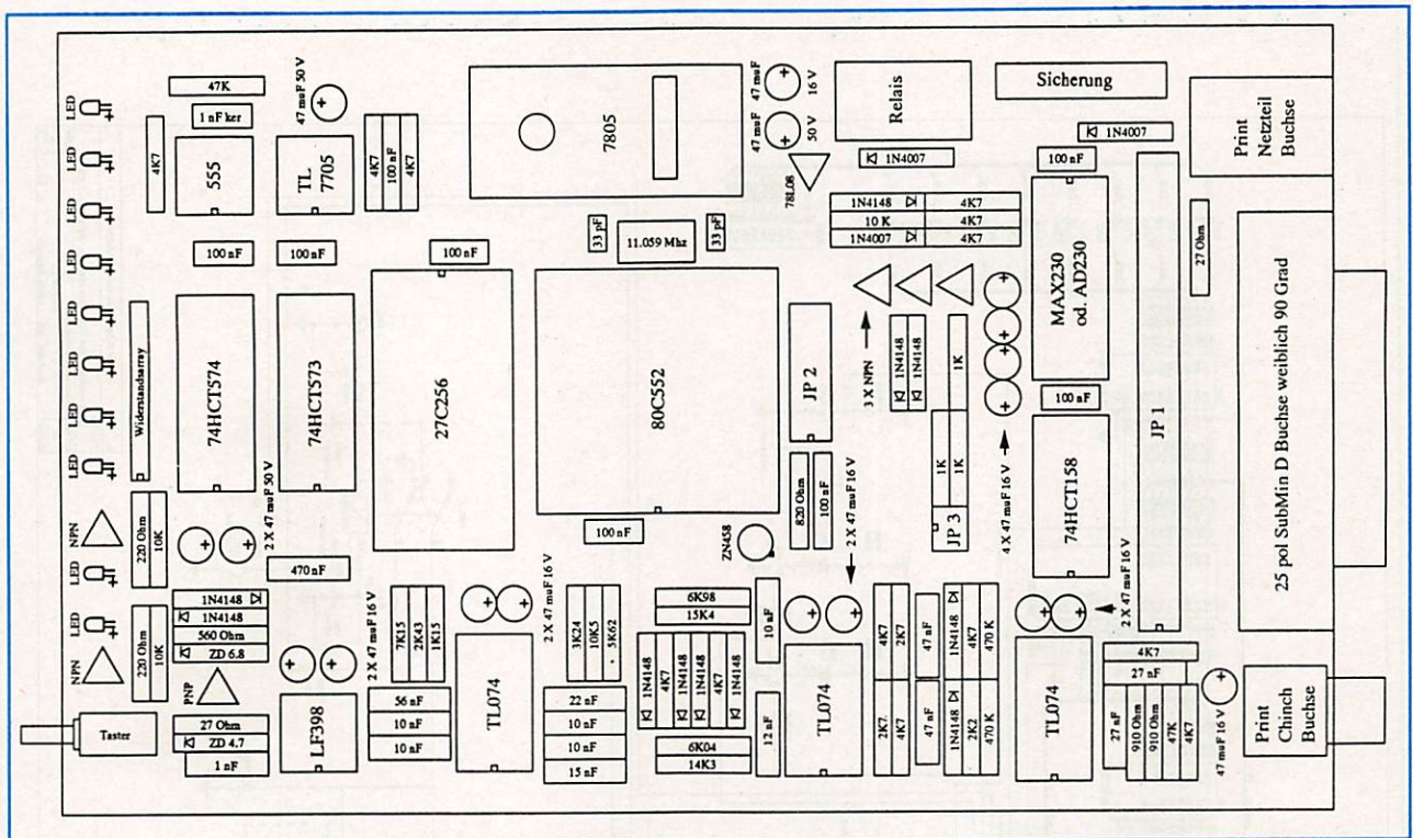
Figure 4 – Schéma d'implantation.
