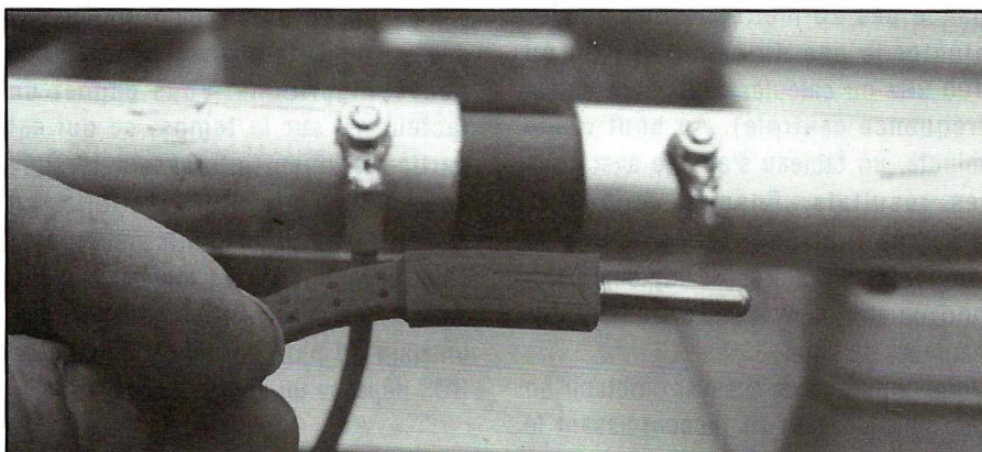
1 La liaison driver est effectuée avec une fiche banane mâle courante. Bien pour l'oxydation et les liaisons HF. Munissez vous de graisse HF.
