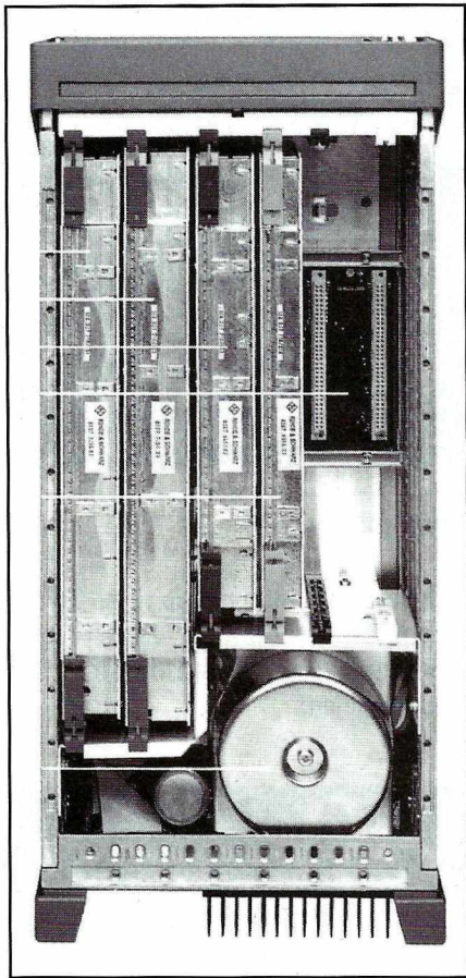
L'intérieur du récepteur : modules enfichables, blindés.
