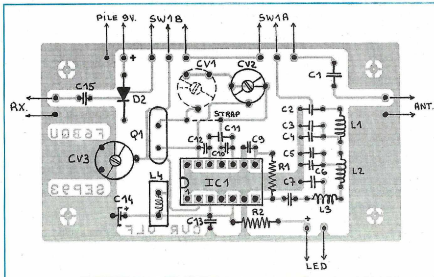
Schéma d'implantation.
