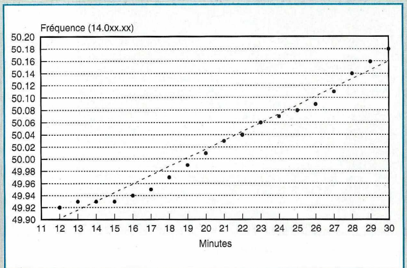
Dérive du VFO.
