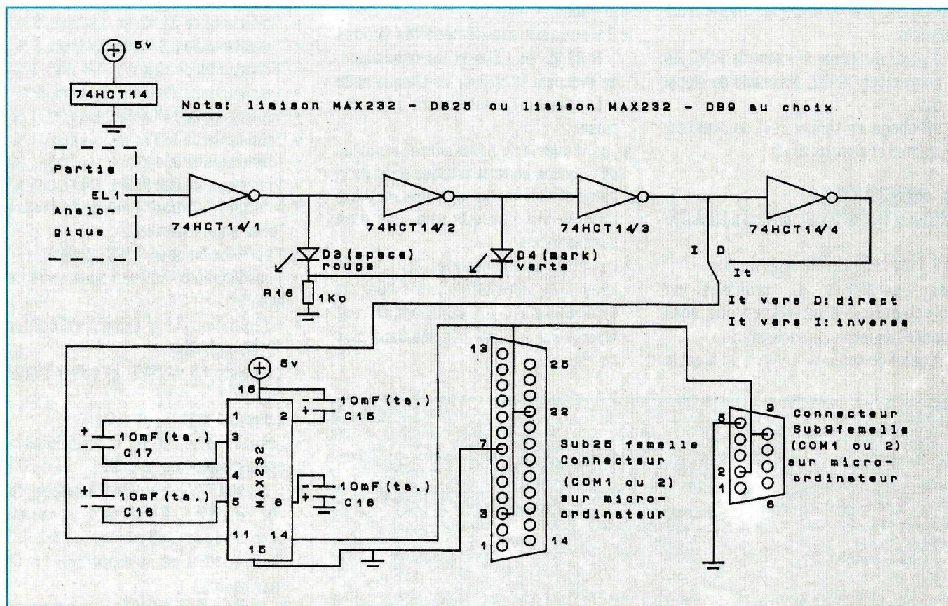
SCHEMA DE PRINCIPE - PARTIE LOGIQUE
