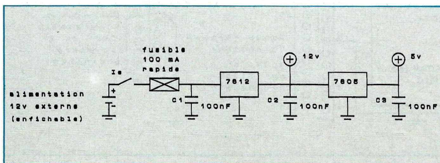
SCHEMA DE PRINCIPE - PARTIE ALIMENTATION
