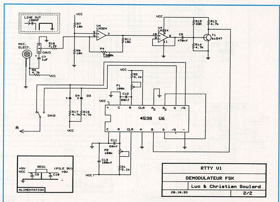
Synoptique.
