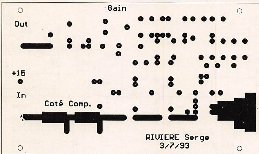
Côté composants
