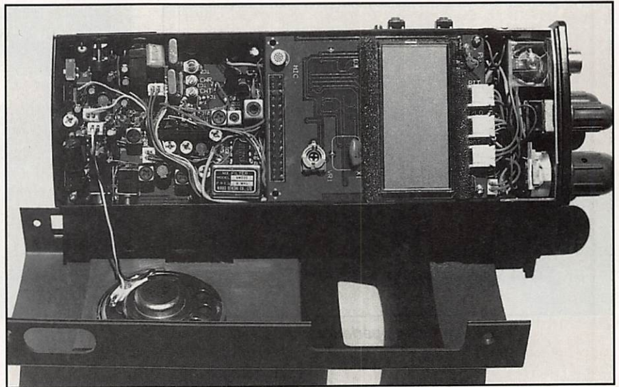
L'afficheur, le synthétiseur et la platine FI.
