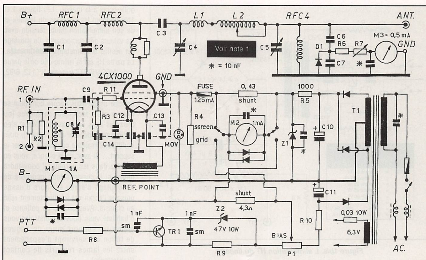
Figure 1. Schéma d'un linéaire "à grille-écran à la masse" muni d'un tube 4CX1000A. Entrée 10 W, sortie 1500 W.
