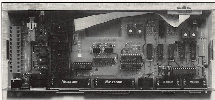
Sur cette vue interne, on aperçoit le bornier, les relais et les « trimers » de pré-réglage.
