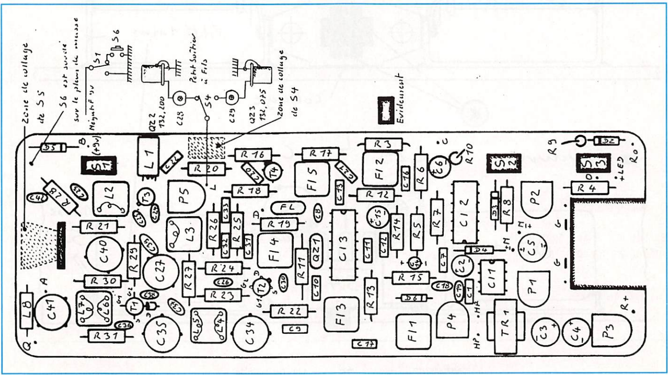
Schéma d'implantation.
