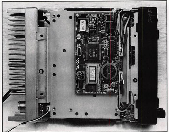
Le DTR-192 côté TNC.
