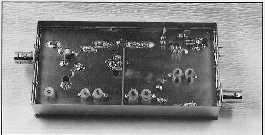
Convertisseur ATV 70 cm, côté plan de masse.
