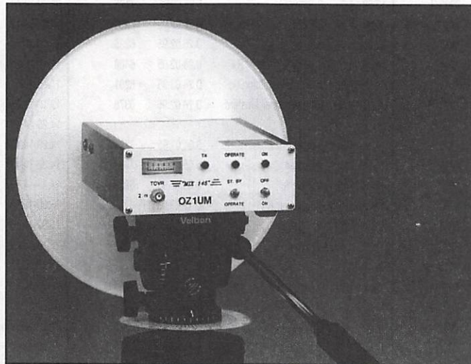
Transverter 145 GHz
