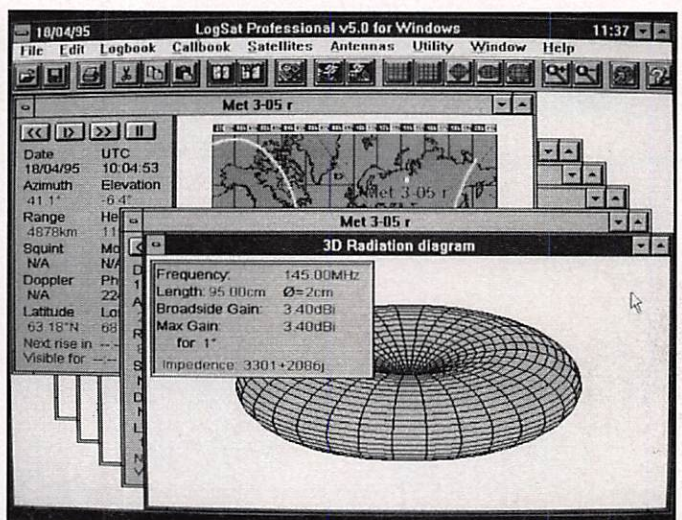
Diagramme de rayonnement d'un dipôle vertical.
