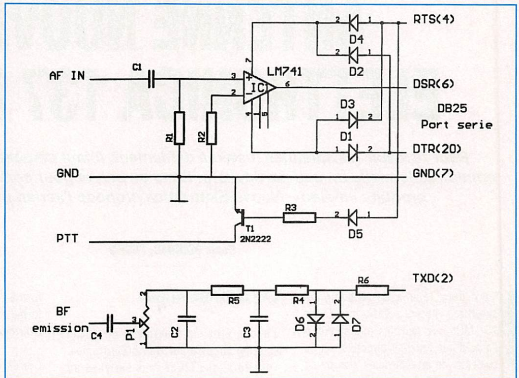
Le schéma de l'interface.
