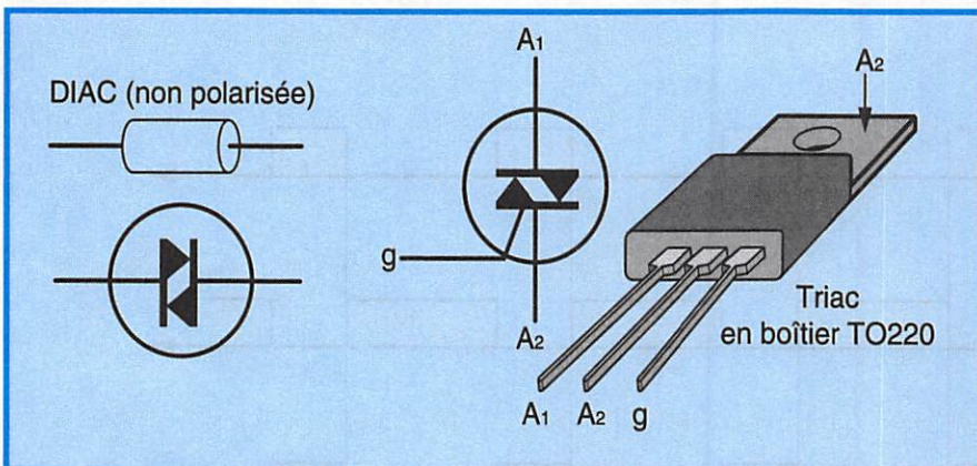
Figure 3. Le brochage des semi-conducteurs.
