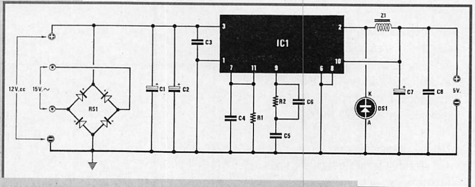
Figure 5. Le schéma de l'alimentation.
