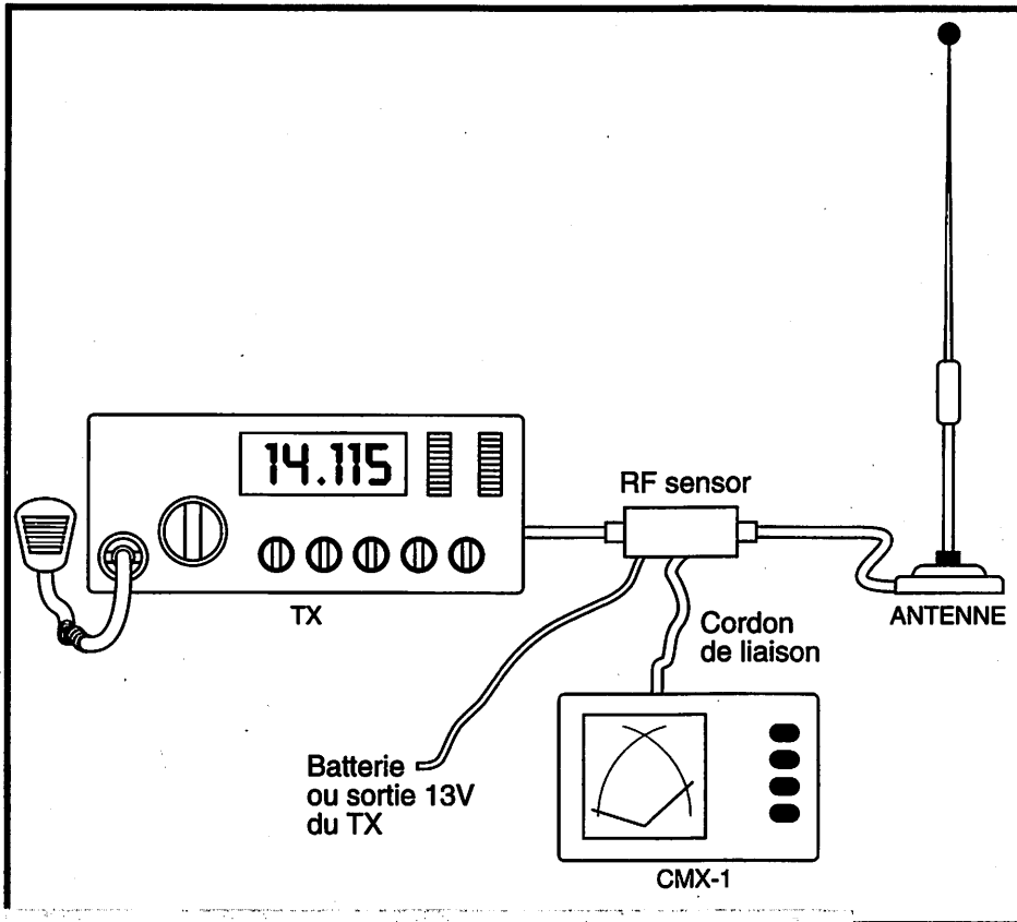
Montage du CMX-1 dans la ligne antenne.
