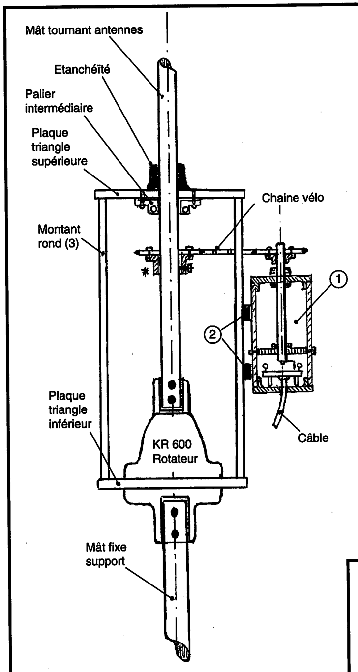
Planche 1. Vue d'ensemble. Positionnement du capteur sur la cage triangulaire du pylône.
