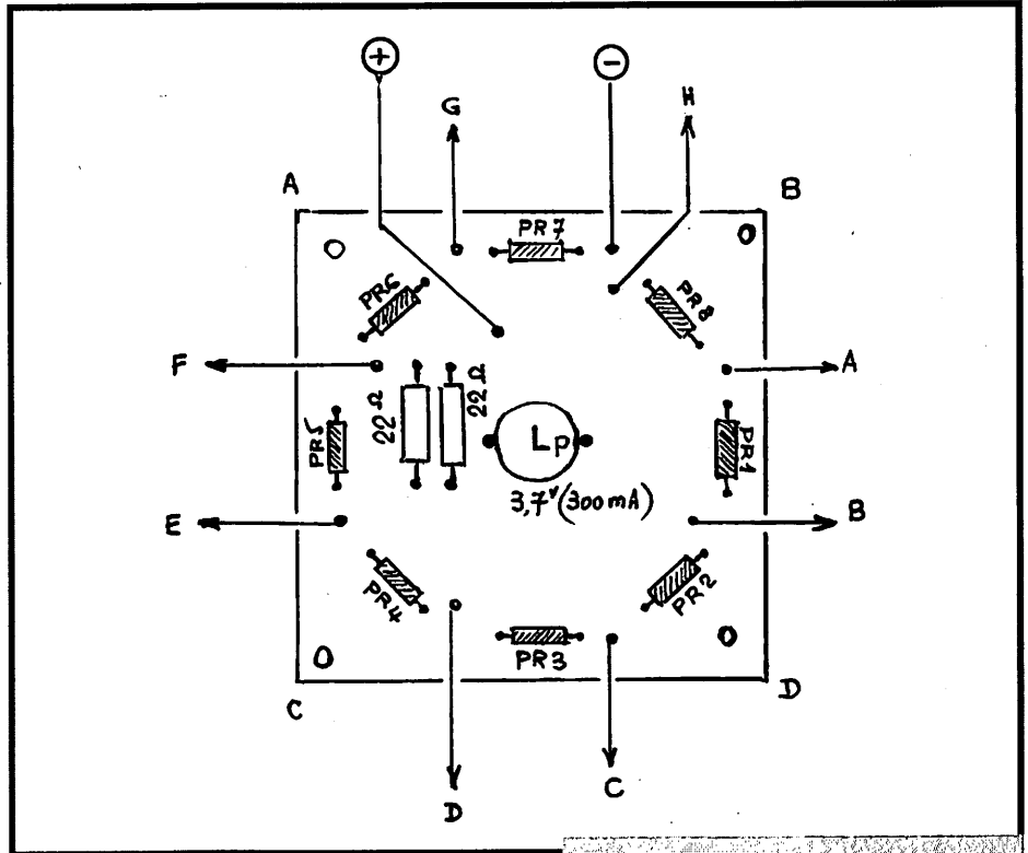
Figure 5. Circuit capteur.
