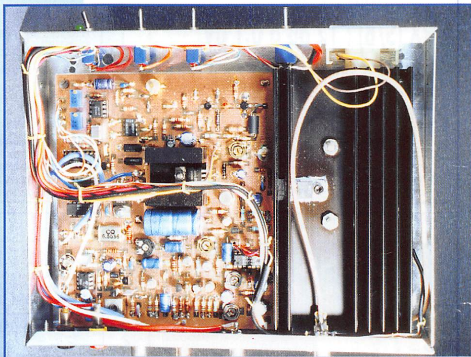
L'intérieur de l'émetteur ATV. Un câblage quasi professionnel.
