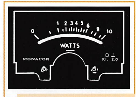
Mylar du cadran (éch. 1).
