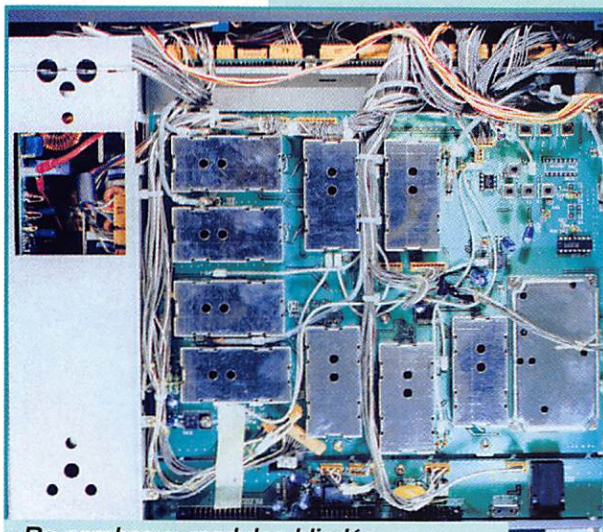
De nombreux modules blindés soudés sur une grande carte.
