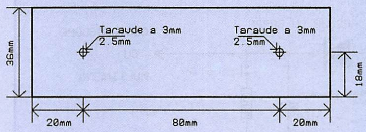
Radiateur SK133
