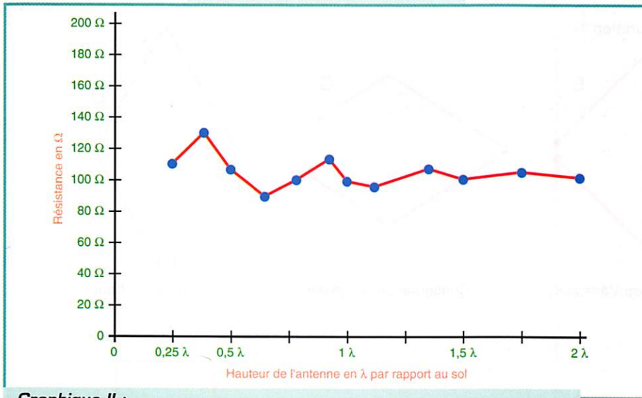
Graphique II : Impédance d'un cadre x ou + par rapport au sol.
