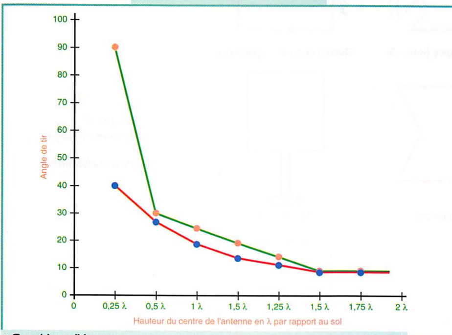
Graphique IV : Angle de tir selon la hauteur au dessus du sol.
