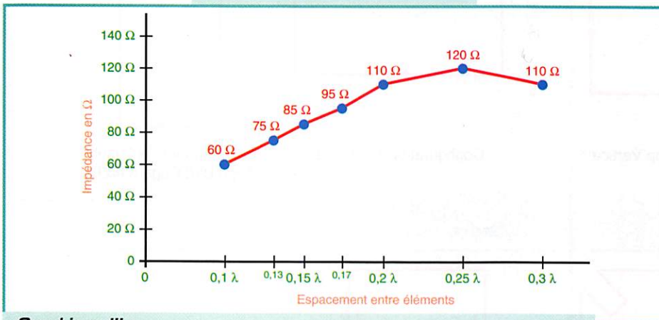
Graphique III : Impédance d'un cadre selon l'espacement d'un élément parasite.
