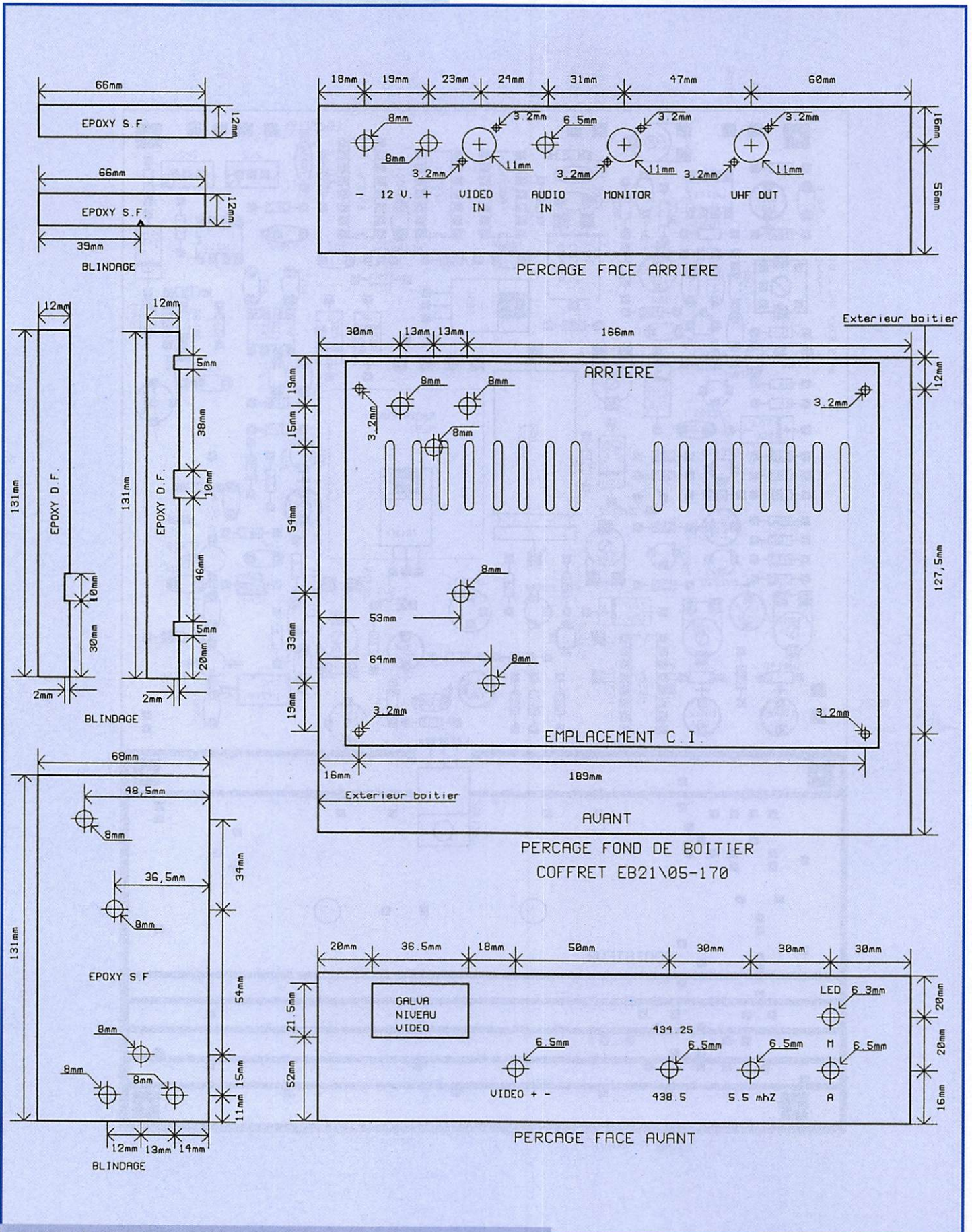
Figure 5. Plan de découpe blindage et de perçage boîtier.
