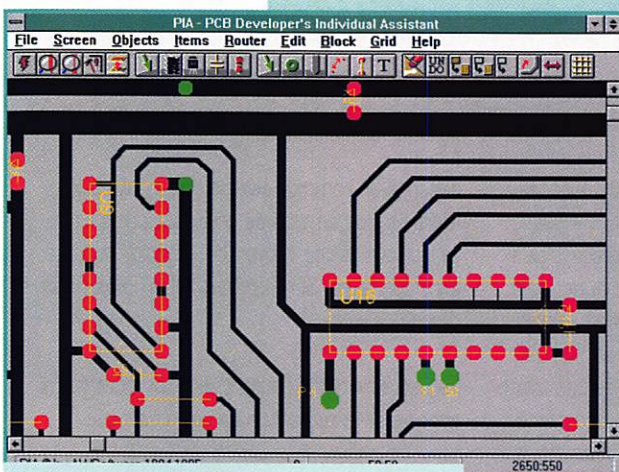
PIA-PCB.
