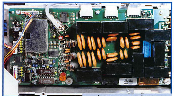
Les commutations vers les deux prises antennes.
