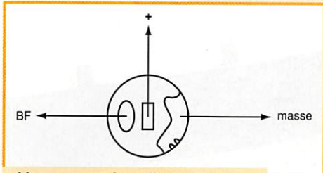
Une connexion d'un micro à électret à 3 sorties.
