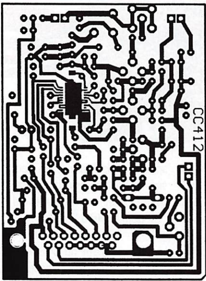
Circuit imprimé face soudures.
