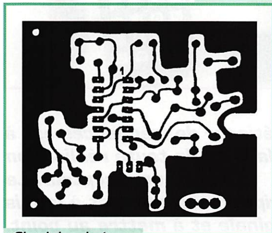
Circuit imprimé, échelle 1.
