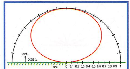
Figure 1-6-c : Diagramme de rayonnement dans le plan vertical d'un doublet demi-onde, fil horizontal placé à 0,25 \lambda du sol.
