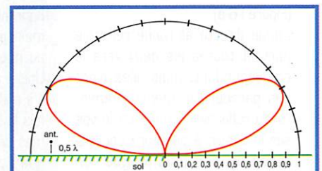
Figure 1-6-d : Diagramme de rayonnement dans le plan vertical d'un doublet demi-onde, fil horizontal placé à 0,5 \lambda du sol.
