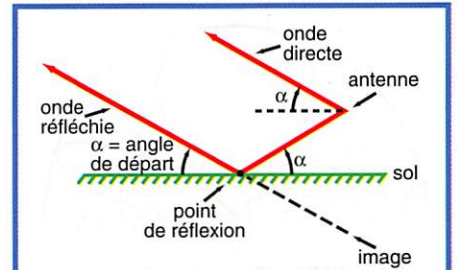
Figure 1-6-a : Réflexion de l'onde sur le sol, et création d'une antenne image. L'onde réfléchie par le sol semble provenir de l'antenne image.
