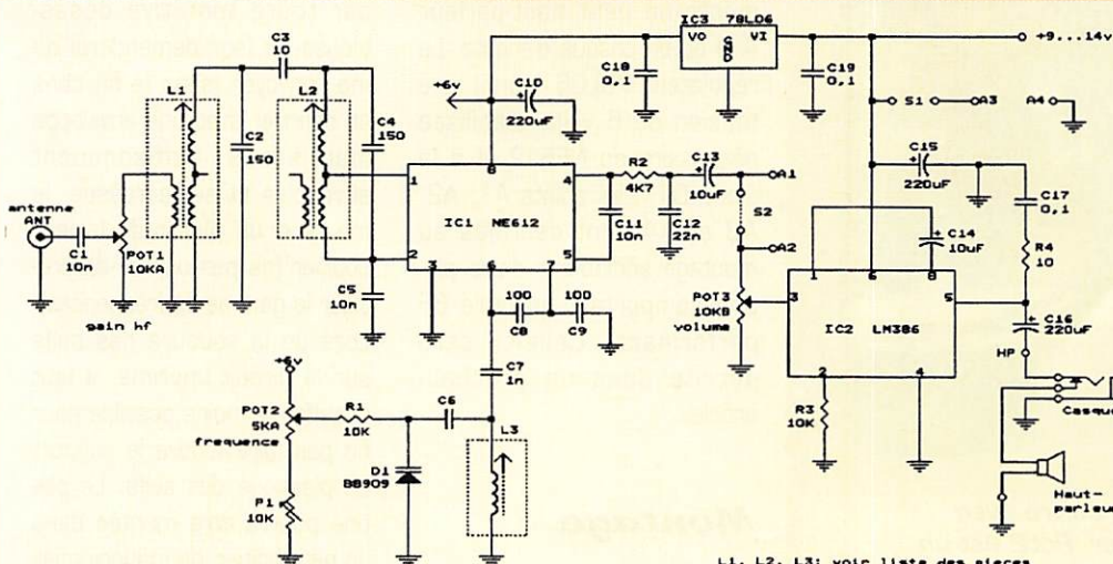
L1, L2, L3: voir liste des pièces C6: voir liste des pièces
