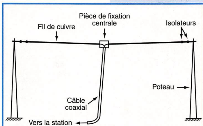
Figure I-7-2-a : Doublet demi-onde suspendu entre deux supports.
