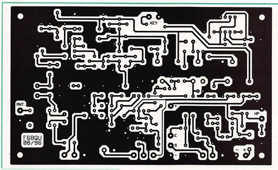
Circuit imprimé.
