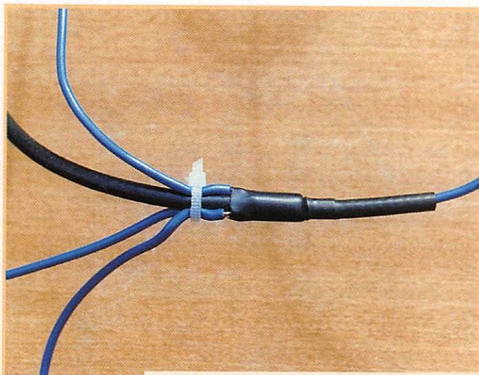
La jonction entre les radians, le brin rayonnant et le coaxial.
