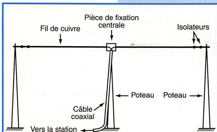
Figure I-7-2-b : Doublet demi-onde monté sur trois supports.
