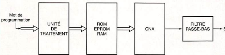
Figure 5 : Synoptique d'un système DDS simple.
