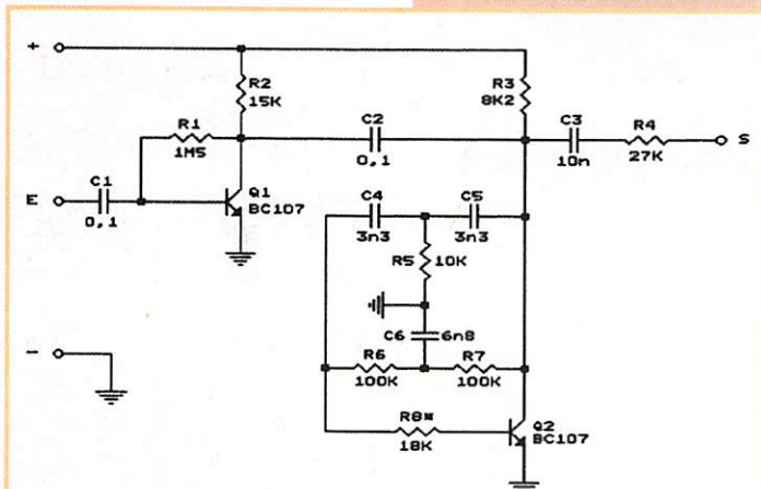
Figure 1 : Filtre BF à transistors.
