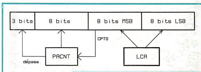
Figure 4 Résultat binaire du comptage.
