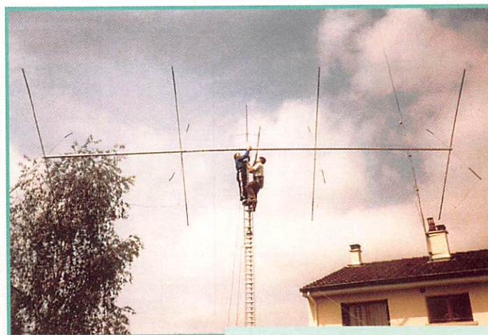
4 éléments quad 21 MHz. Antenne F6DPR, F6DDR.
