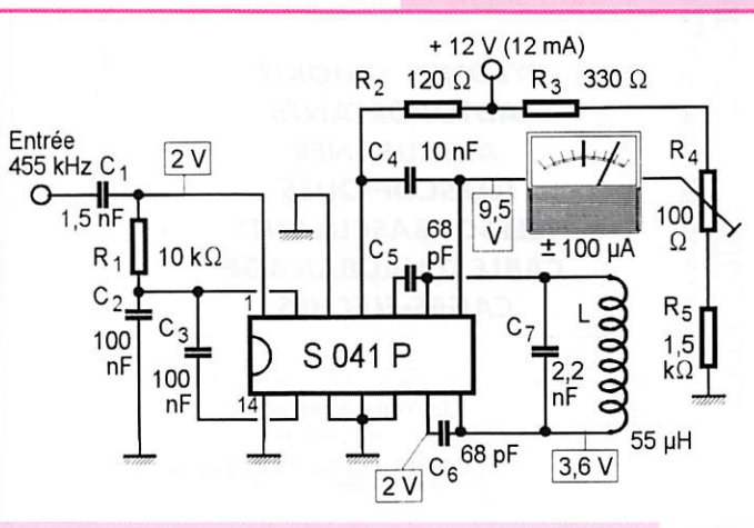
Fig. 1. — L'indicateur d'accord utilise un démodulateur pour modulation de fréquence, transformant tout écart de fréquence en une tension proportionnelle. Les tensions indiquées sont les valeurs continues de repos.
