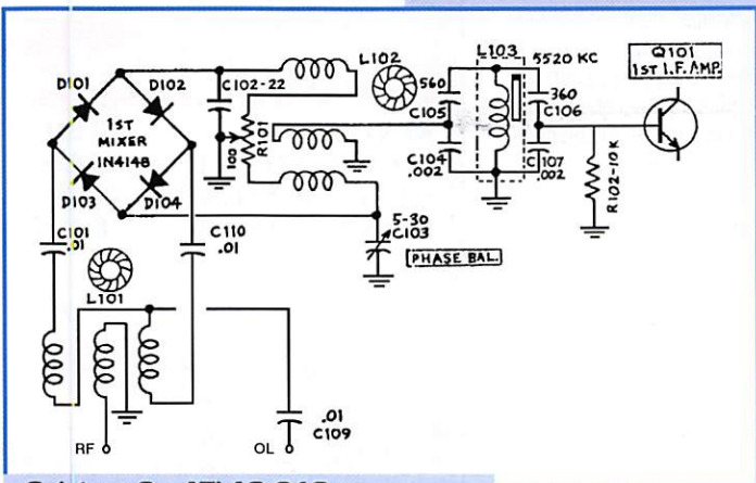
Schéma 8 : ATLAS 210. Mélangeur HF.
