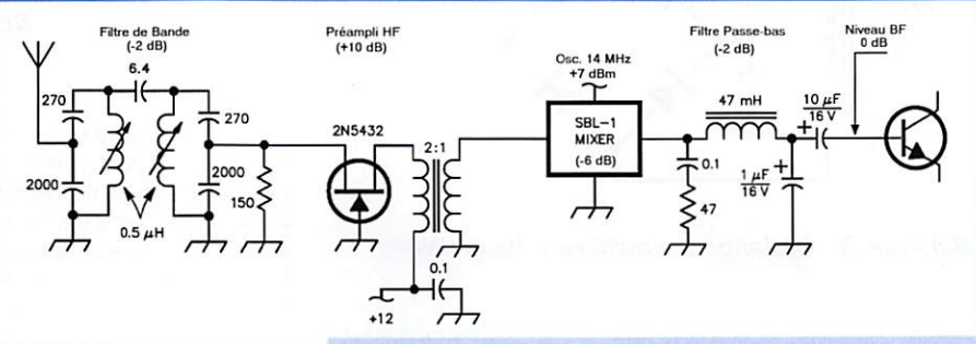
Schéma 9 : Récepteur à conversion directe (bande 14 MHz).
